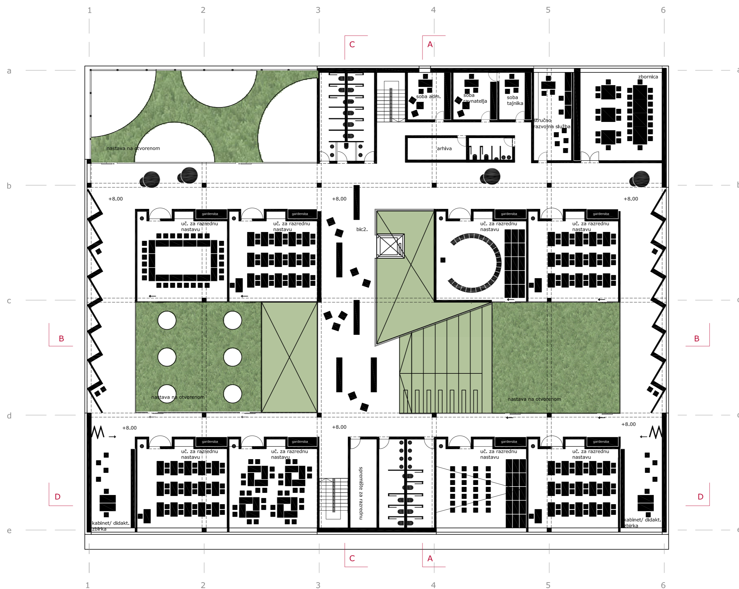
TLOCRT 2. KATA
