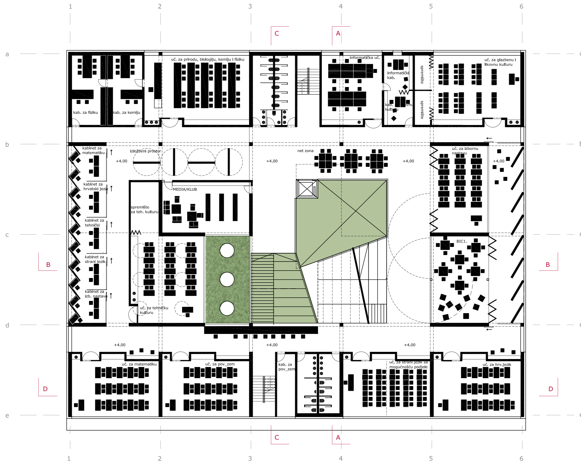
TLOCRT 1. KATA
