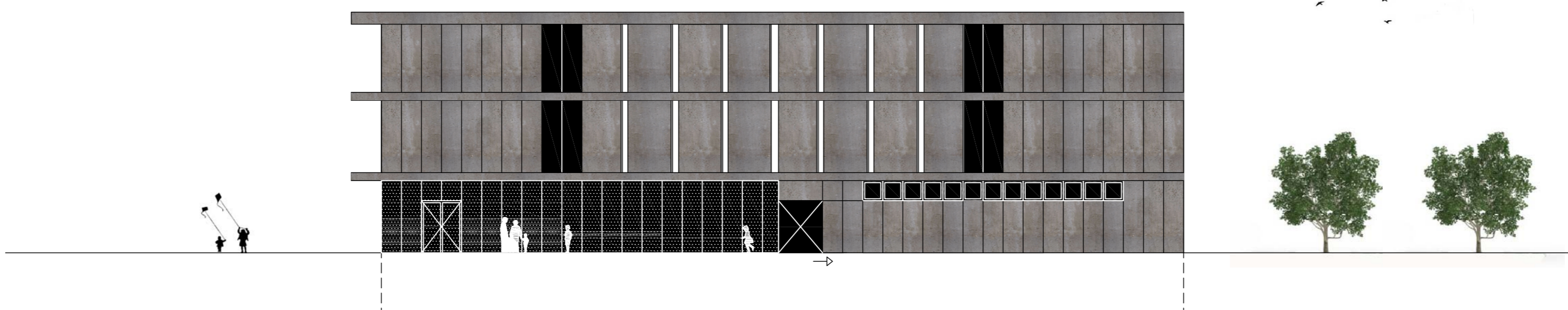
ISTOČNO PROČELJE
