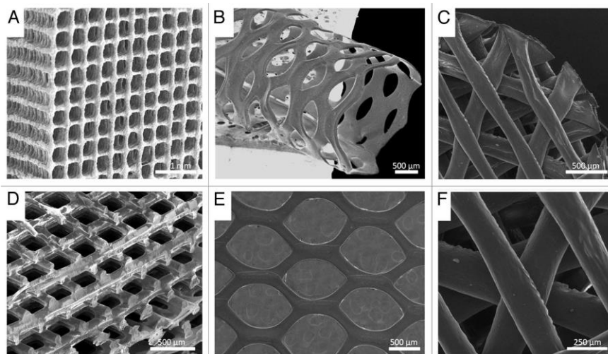
Slika 9. Različiti oblici mrežica (eng. scaffold ); A- ortogonalni, B- cjevasti heksagonalni plašt, C- ortogonalni, D-ortogonalni, E- heksagonalni plašt, F- dijagonalni [36].
