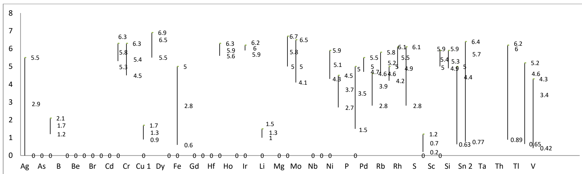
Slika 17. Grafički prikaz raspodjele uzorka metalnih iona na razvijenim kromatografskim pločicama 48 do 55
