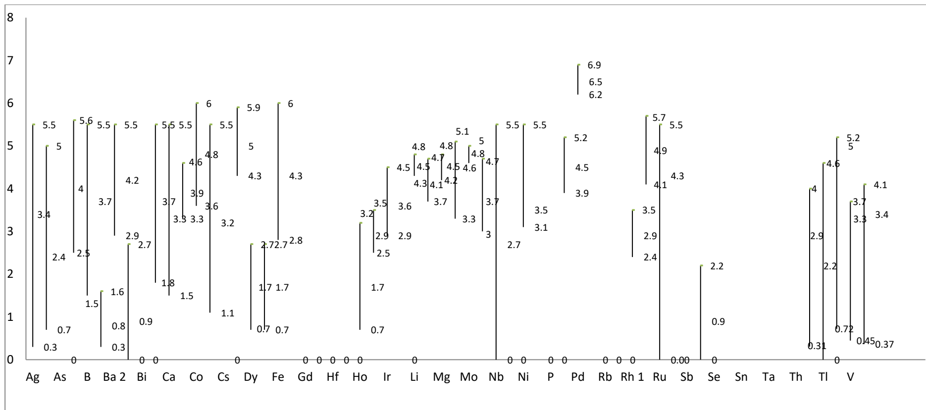
Slika 18. Grafički prikaz raspodjele uzoraka metalnih iona na razvijenim kromatografskim pločicama 56 do 63.
