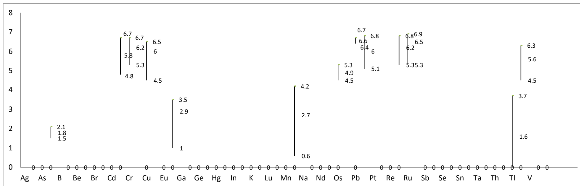
Slika 16. Grafički prikaz raspodjele uzoraka metalnih iona na razvijenim kromatografskim pločicama 40 do 47
