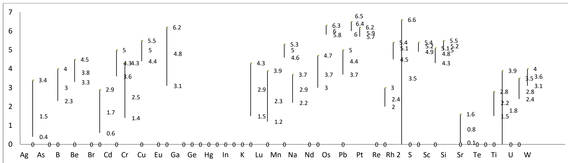
Slika 15. Grafički prikaz raspodjele uzoraka metalnih iona na razvijenim kromatografskim pločicama 32 do 39
