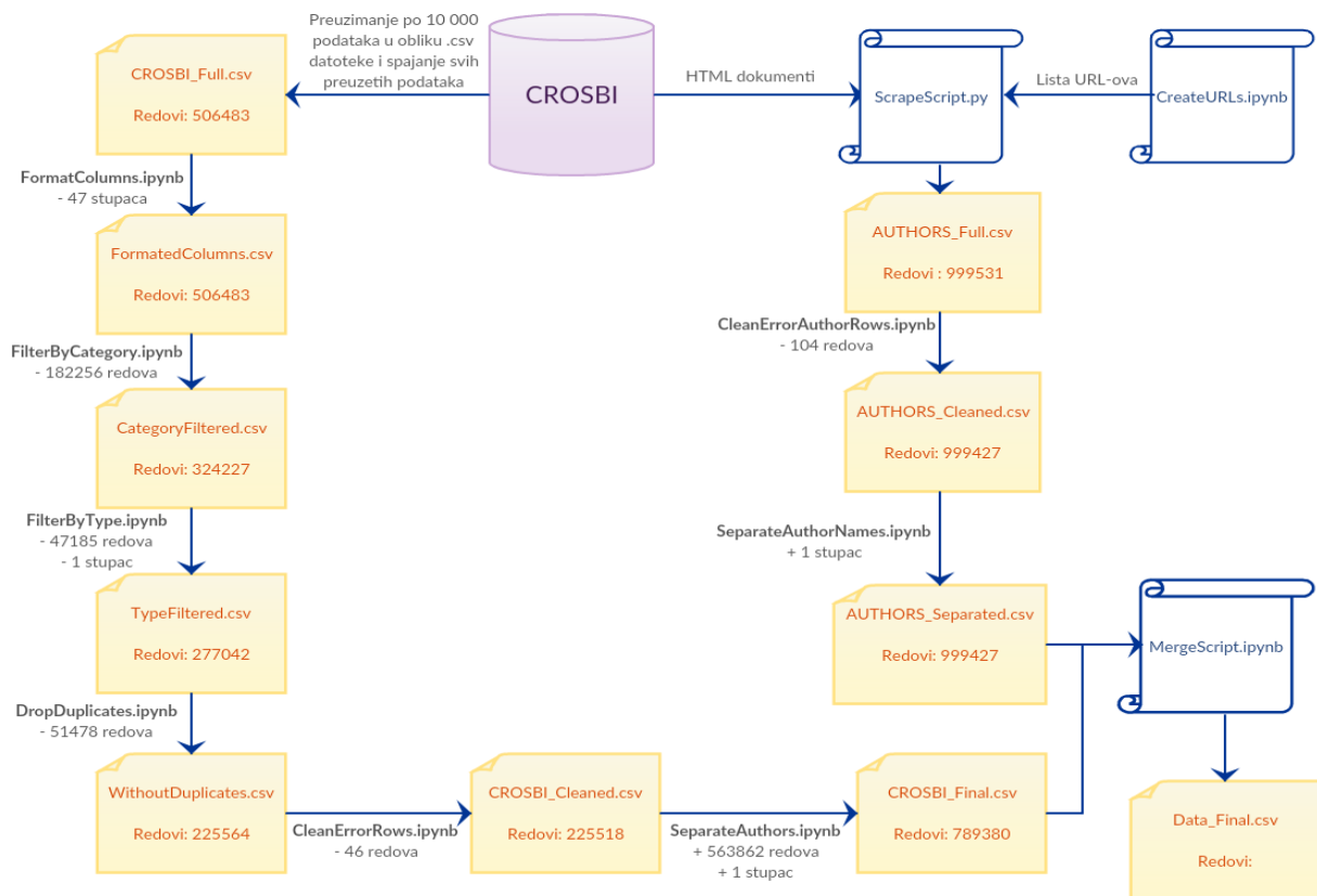
Slika 6. Dijagram transformacije podataka (Samostalna izrada, 2019)
