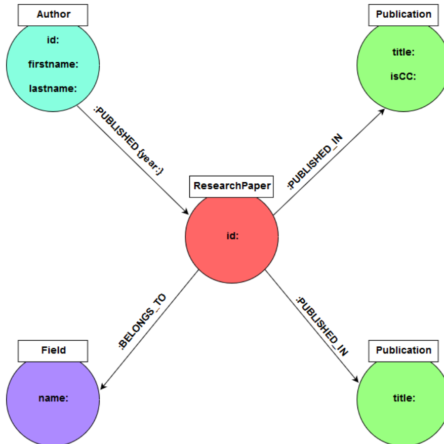
Slika 9. Model podataka grafovske baze podataka (izrada autora)
